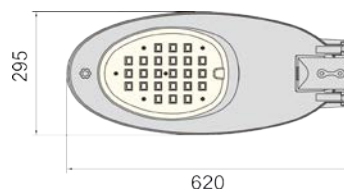
Размеры для монтажа
