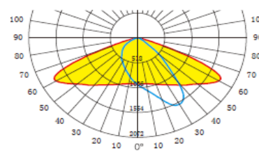
Кривая силы света
