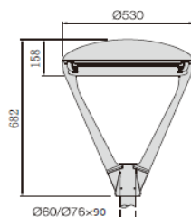
Размеры для монтажа
