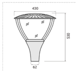
Размеры для монтажа
