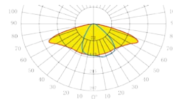
Кривая силы света
