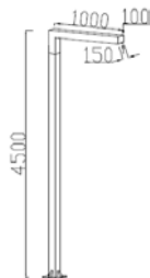
Размеры для монтажа
