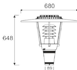
Размеры для монтажа
