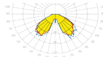
Кривая силы света
