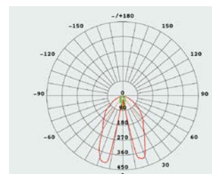
Кривая силы света
